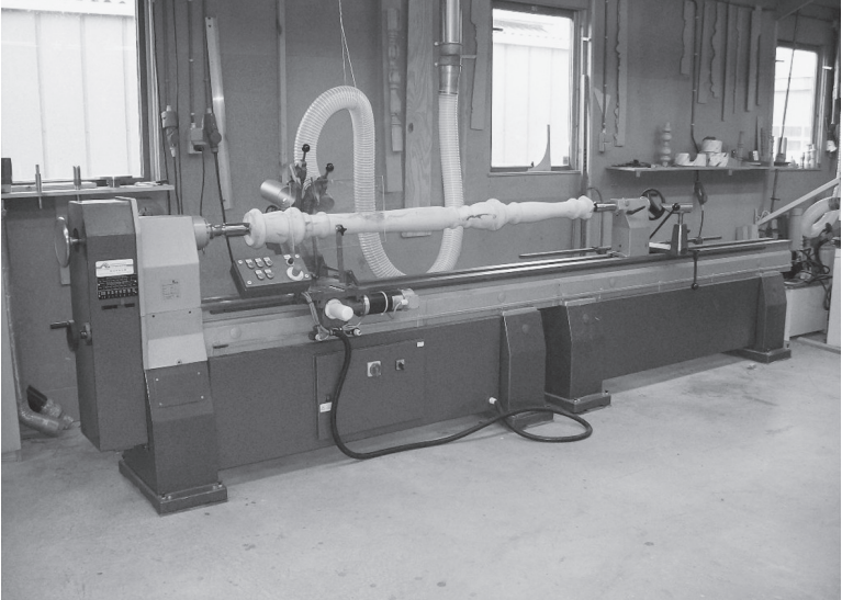
De grootste draaibank van het noorden. (eigen foto)
