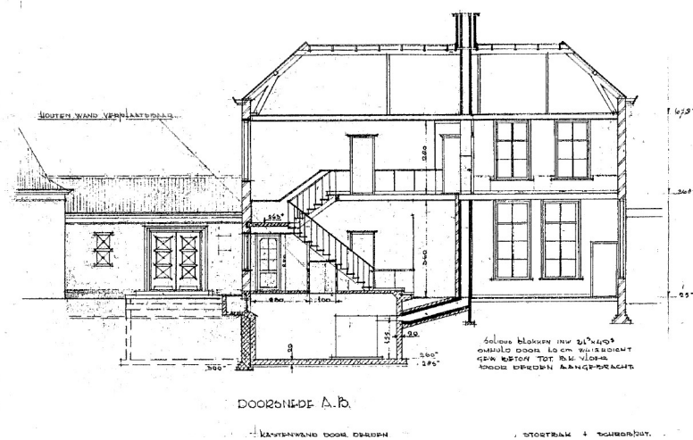
Een onderdeel van het bouwplan voor de verbouwing van 1953
