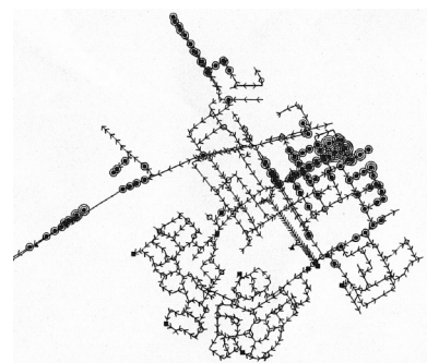
De rioolafvoerpunten in het stratenplan van Buitenpost. Waar cirkels ingetekend staan is sprake van grotere belasting.
