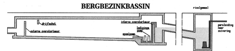
Een overzicht van de onderdelen van de bassin. Links op de tekening staat de afvoer in verbinding met de Buitenposter Vaart. Rechts is de Kuipersweg-kant.
